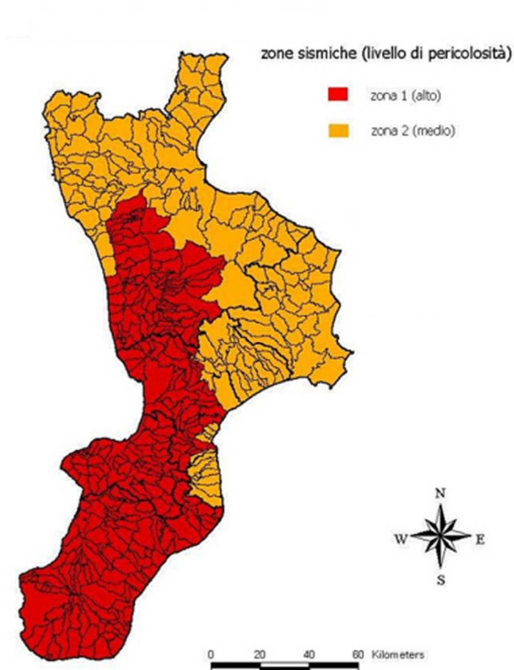
Figura 74: Il rischio sismico in Calabria
